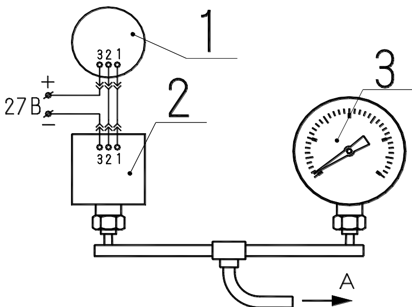
Рисунок 6 - Схема определения основной погрешности:
