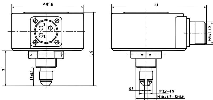
Рисунок 2 - Габаритные и присоединительные размеры приемника
