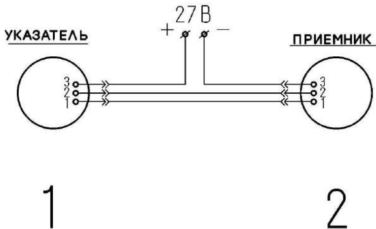
Рисунок 4 - Электромонтажная схема соединения
